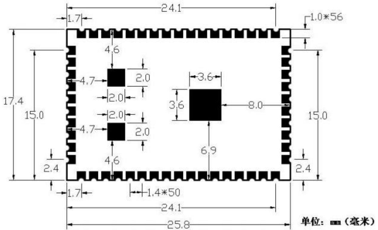
HLK-RM08S 尺寸图
